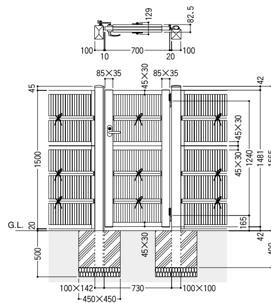
● 寸法図 (単位mm) 清水垣門扉 片開き門柱式 (右勝手内開き) NDS042H
