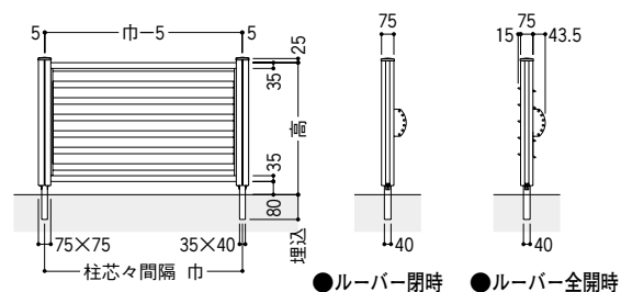
●寸法図 (単位mm) 高:800
