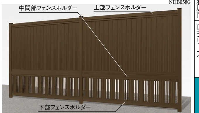
間柱式 上段2N型 高:1200+下段6N型 高:600の組合せ [CBブラウン]
